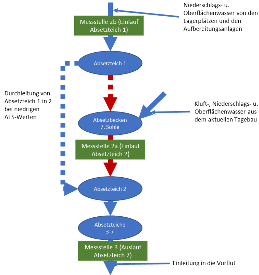
Schema Wasserhaltungskonzept Diabaswerk Huneberg (aktuell)
