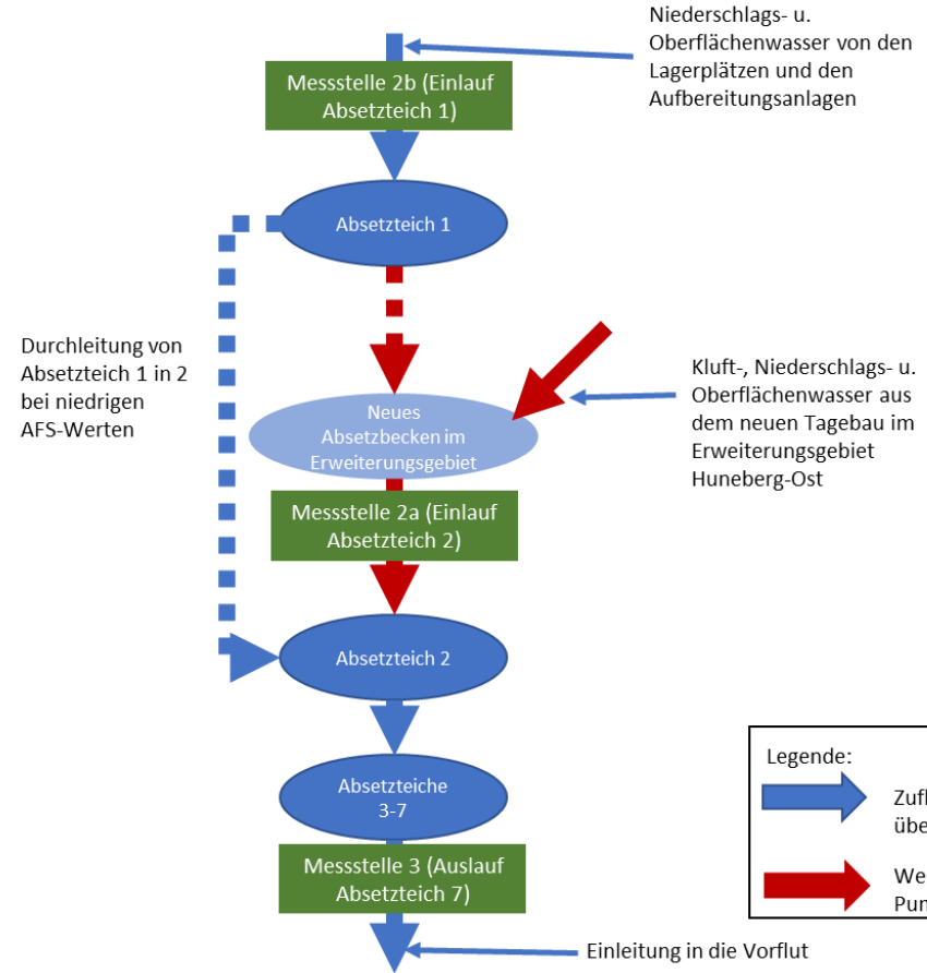
Schema Wasserhaltungskonzept Diabaswerk Huneberg und Huneberg-Ost (geplant)
