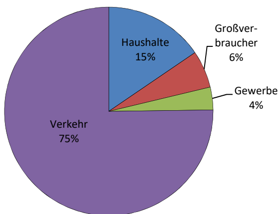
Treibhausgas-Emissionen nach Sektoren
