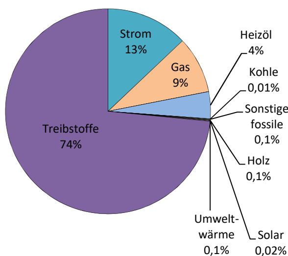
Treibhausgas-Emissionen nach Energieträgern
